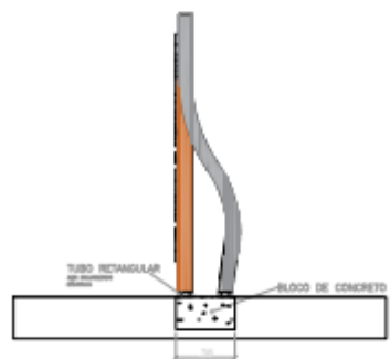
5 Corte 01
