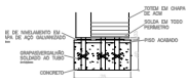
4 Fundação
